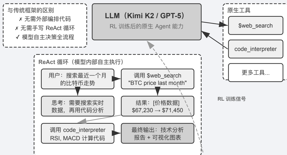
图 1-4：“模型即 Agent”架构——原生工具调用
