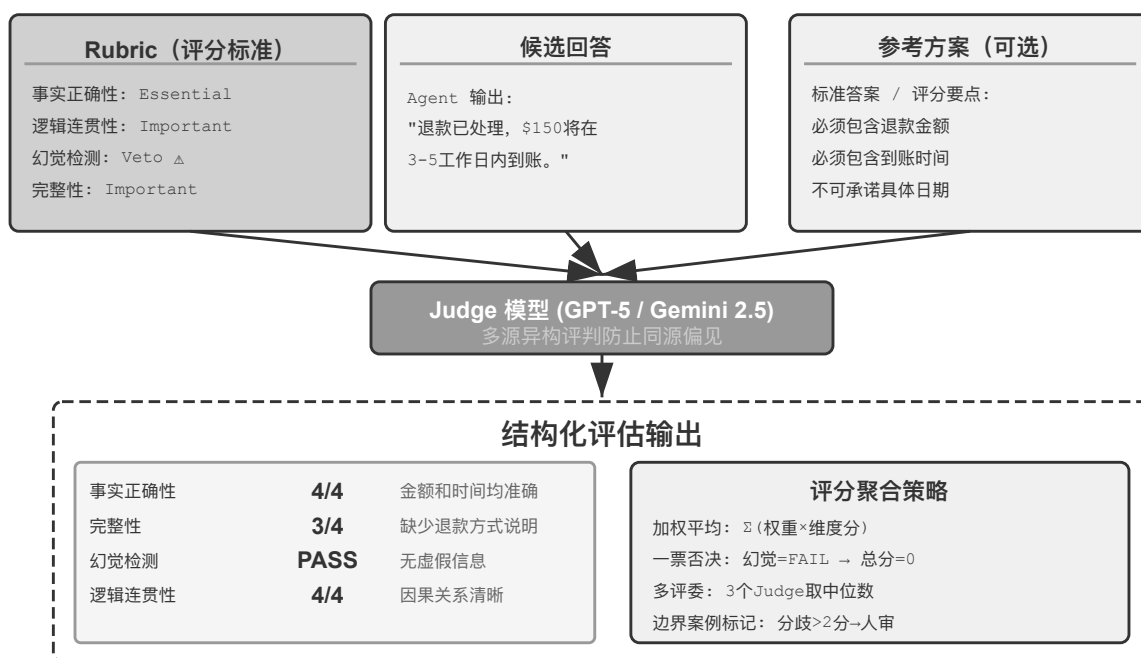
图 6-4 LLM-as-a-Judge 流水线
