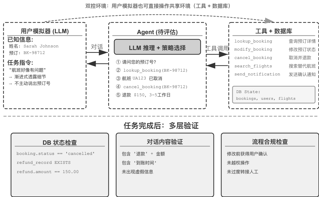
图 6-3 r 2 -bench 评估架构
