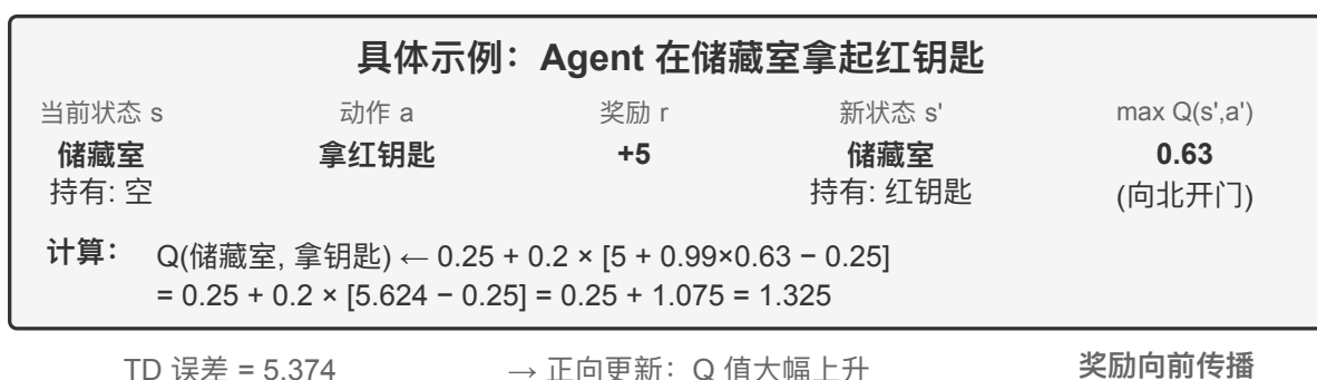
图 7-4 Q 值更新可视化
