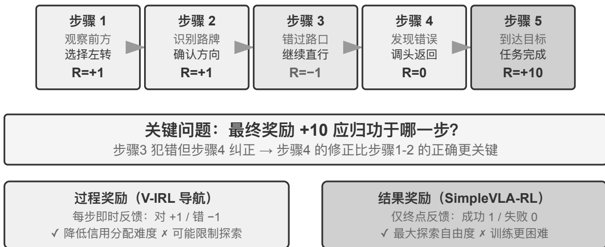
图 7-15 多轮交互中的信用分配
